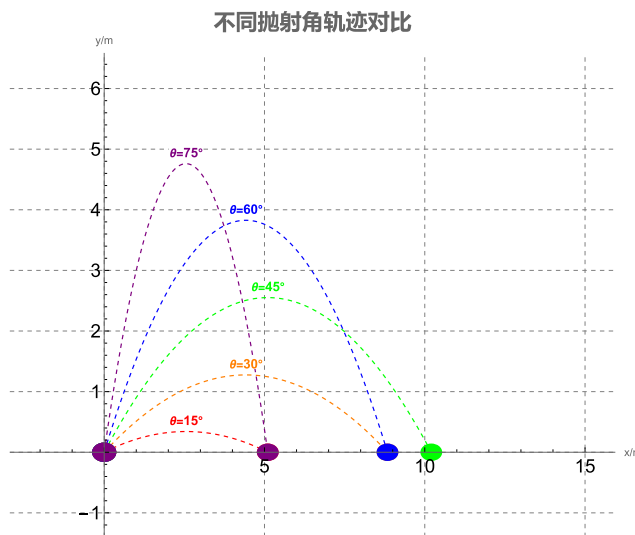
图 2 不同抛射角度下斜抛运动轨迹对比图
