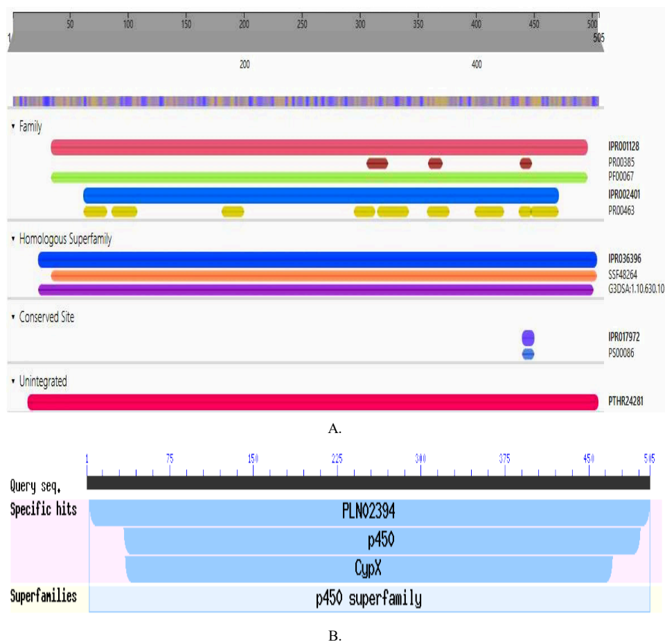
图 4 蛋白序列的保守结构域分析。A. InterProScan 分析结果, B. GeneBank 的 Conserved domains 分析结果。
