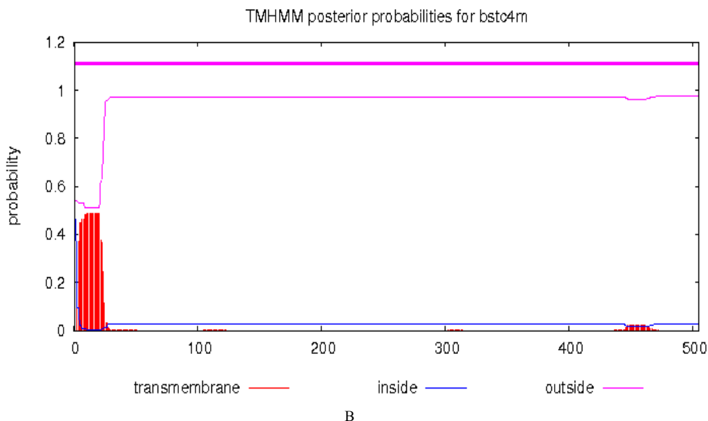
图 6 BsC4H 蛋白的亚细胞定位分析。A. 信号肽预测, B. 跨膜结构域分析。
