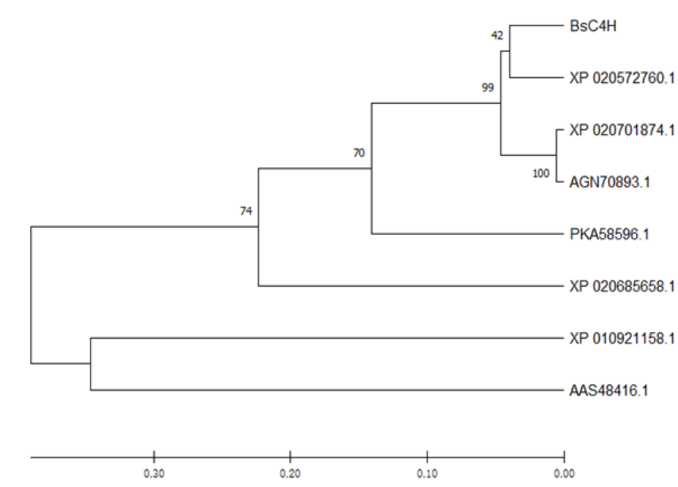
图 3 氨基酸序列进化树分析
