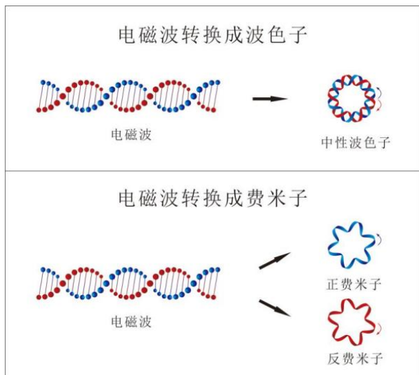
图4 粒子转换过程
