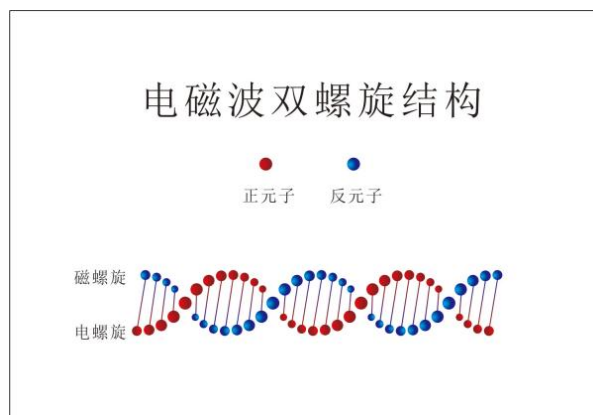
图2 双螺旋结构
