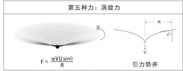
图9 涡旋力
