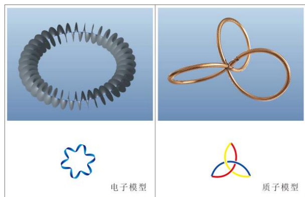
图5 电子质子模型
