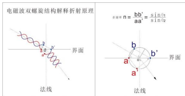
图3 折射原理
