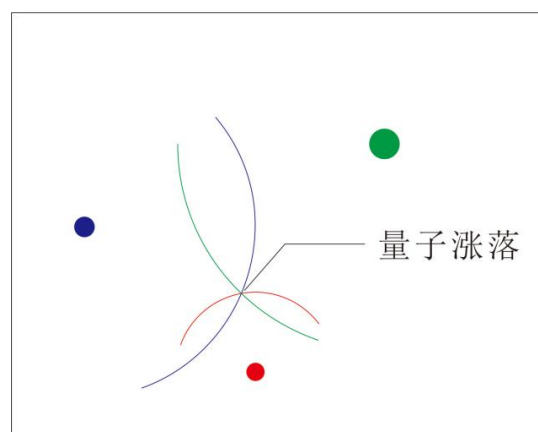
图1 真空量子涨落
