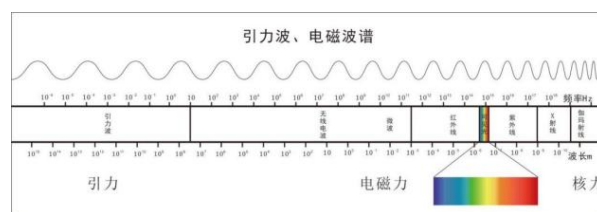
图 8 波谱
