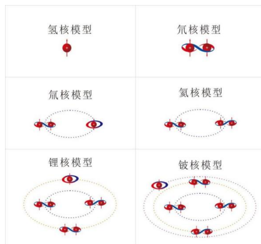
图6 原子核模型
