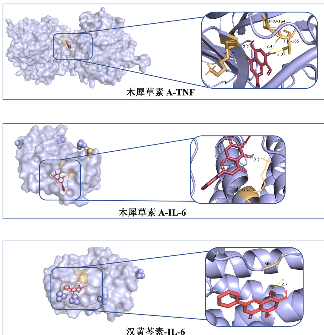
图 7 IL-6、TNF 与穿心莲化合物的最佳分子对接模式
