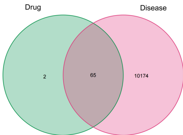
图 1 穿心莲-COPD 靶点交集韦恩图
